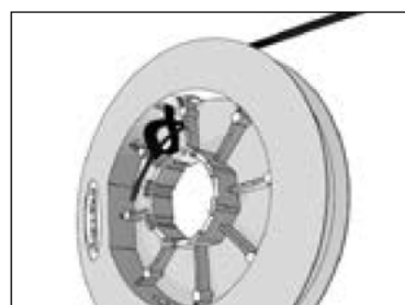
Протяните ленту (шнур, корд) из лентоукладчика (укладчика шнура или корда) в отверстие для вывода элементов управления. Закрепите ленту на шкиве, завязав узел.
