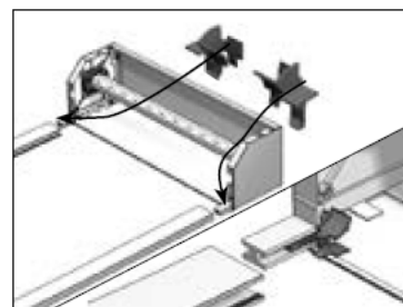
Установите направляющие устройства в пазы боковых крышек.
