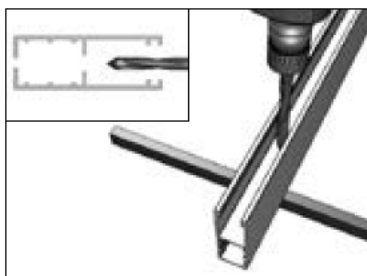
Вариант встроенного монтажа Просверлите отверстия \varnothing 8 мм в направляющих шинах через внутренние стенки. Рассверлите отверстия во внутренней стенке направляющей шины под шляпки саморезов \varnothing 12 мм или \varnothing 14 мм в зависимости от комплектации.
