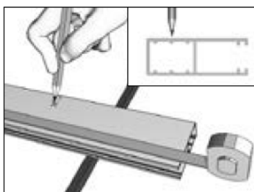
Вариант накладного монтажа Нанесите отверстия на направляющих: центры отверстий должны располагаться по центру относительно паза в направляющей.
