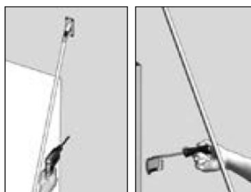
Наметьте и просверлите отверстия для крепления клипсы (при ее наличии в комплектации). Закрепите клипсу саморезами.
