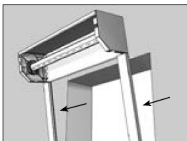
Снимите каркас роллеты с места монтажа.
