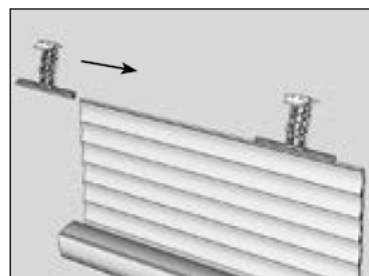
Вариант монтажа роллеты с ригелями Вставьте ригели в верхний профиль полотна.
