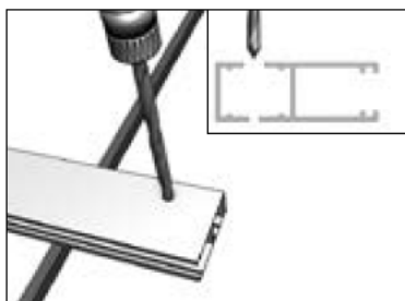
Вариант накладного монтажа Просверлите отверстия \varnothing 8 мм в направляющих шинах через две стенки. Рассверлите отверстия на лицевой поверхности направляющей шины под заглушки \varnothing 12 мм или \varnothing 14 мм в зависимости от комплектации.
