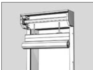
Заправьте тяговые пружины в продольные перфорационные отверстия вала.
