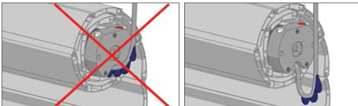
Монтаж кабеля электродвигателя проводить с изгибом согласно рисунку.
