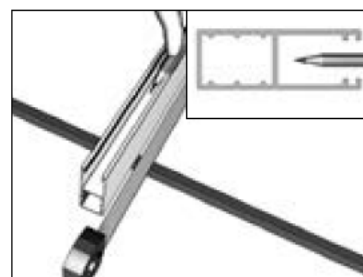
Вариант встроенного монтажа Нанесите отверстия на направляющих: центры отверстий должны располагаться по центру перегородки в направляющей.
