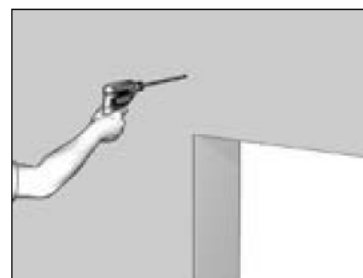
Рассверлите намеченные отверстия в стене для вывода элементов управления: для вывода кабеля электродвигателя, шнура — отверстие \varnothing 12 мм; для вывода ленты — отверстие \varnothing 16-18 мм; для вывода кардана, корда — отверстие \varnothing 14-16 мм; рассверлите отверстие \varnothing 20 мм на необходимую глубину под цилиндрический выступ кардана.
