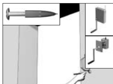
Вариант монтажа роллеты с ленточным, шнуровым или кордовым приводом Разметьте и просверлите отверстия Ø8 мм для установки дюбелей и крепления лентоукладчика (аналогичная операция производится для укладчика шнура или корда).
