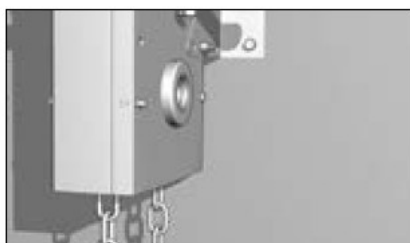
Установите натяжной ролик с фиксатором цепи на высоте 1 м и на одной оси с приводом. Разметьте и просверлите отверстия в стене для крепления натяжного ролика.
