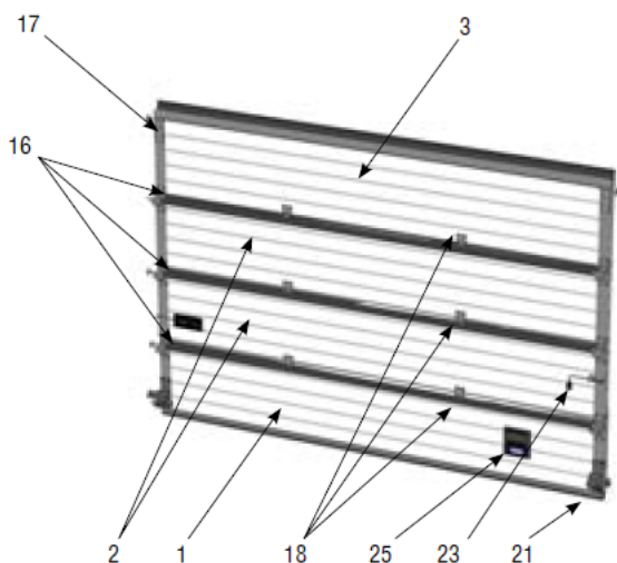
Щит секционных ворот
