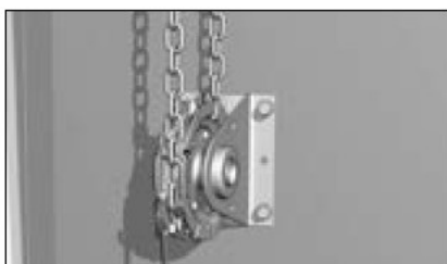
Проденьте цепь через привод и натяжной ролик.
