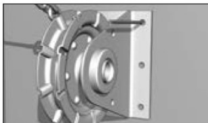
Установите натяжной ролик с фиксатором цепи на высоте 1 м и на одной оси с приводом. Разметьте и просверлите отверстия в стене для крепления натяжного ролика.
