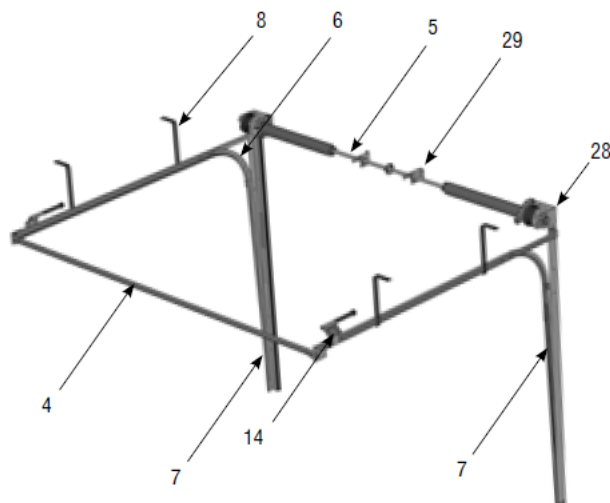
Система направляющих и тормозных механизмов
