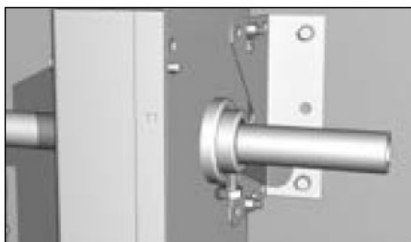
Вставьте дюбель и закрепите кронштейн крепления ручного цепного привода к стене при помощи саморезов и к приводу при помощи шайб с гайками.
